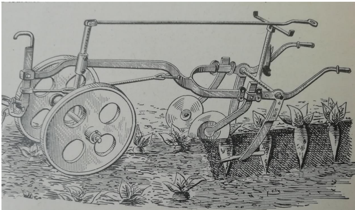
Figure 1: La souleveuse de betteraves. Source : Larousse agricole sous la direction de E. Chancrin et de R. Dumont. Paris. 1921.
